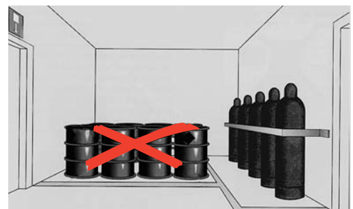
Bild 4: Falsch ist zum Beispiel das Lagern von Gasflaschen mit brennbaren Gasen neben Fässern mit Lösemitteln.
