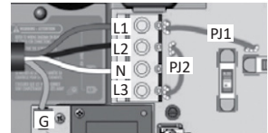
3 Phasen Anschluss Delta
